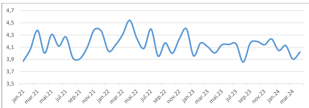
Figur 25 Liggetid sykehusopphold
