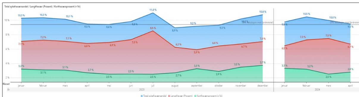
Figur 32 Sykefravær
